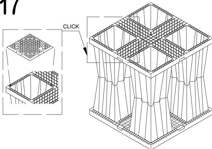
CHIUSURA SUPERIORE AQUABOX
