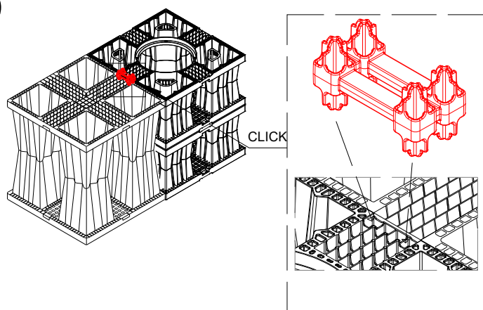
5 CONNETTORE DOPPIO
