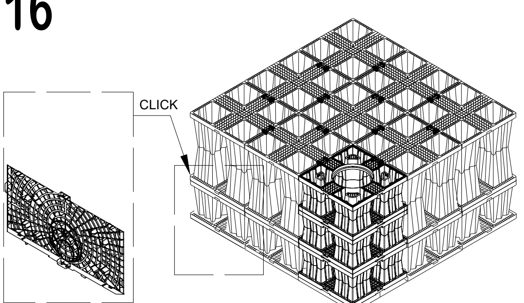
GRIGLIA LATERALE AQUABOX HALF
