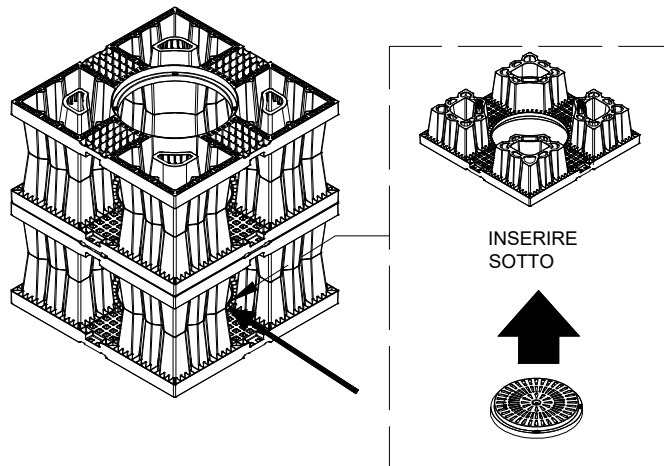
4 COPERCHIO D400
