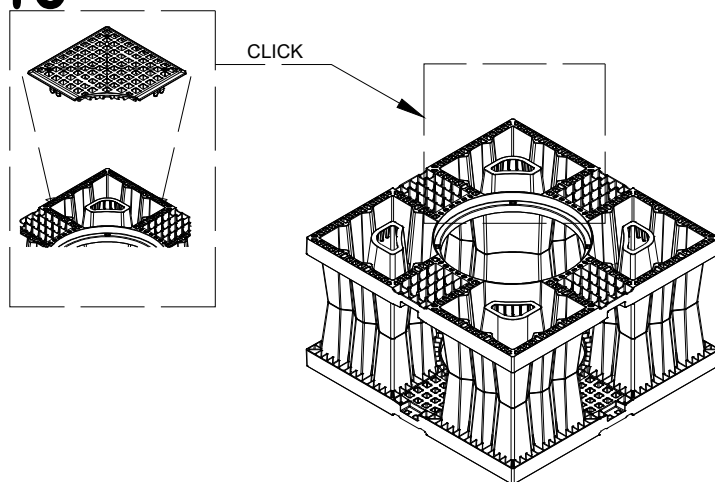
GRIGLIA LATERALE AQUABOX
