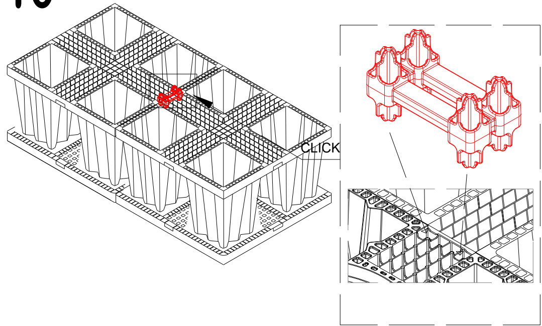
CONNETTORE DOPPIO
