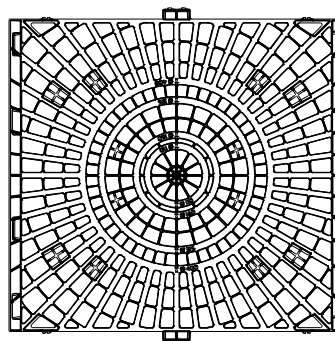
GRIGLIA LATERALE AQUABOX
