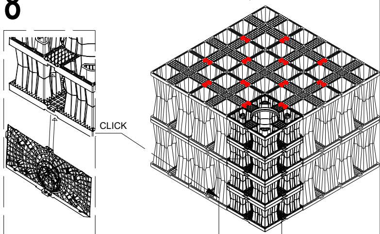
8 GRIGLIA LATERALE AQUABOX CUBE
