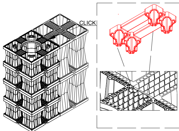
7 CONNETTORE SINGOLO
