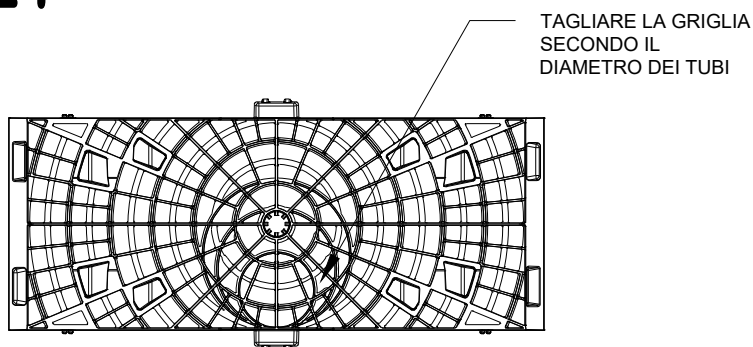
GRIGLIA LATERALE AQUABOX CUBE
