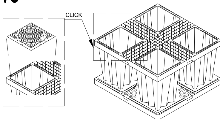
CHIUSURA SUPERIORE AQUABOX
