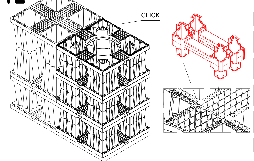
CONNETTORE SINGOLO
