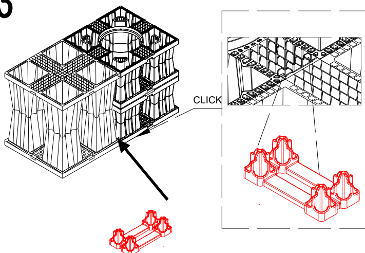
5 CONNETTORE DOPPIO
