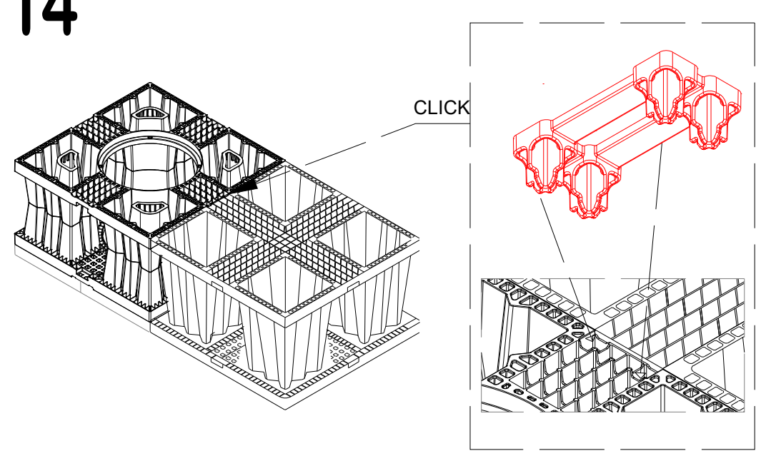
CONNETTORE SINGOLO
