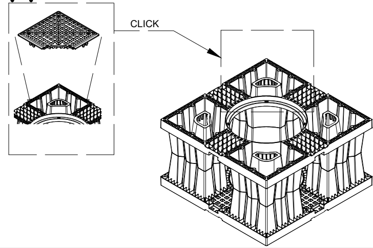
CHIUSURA SUPERIORE AQUABOX
