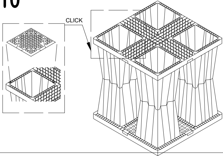
GRIGLIA LATERALE AQUABOX
