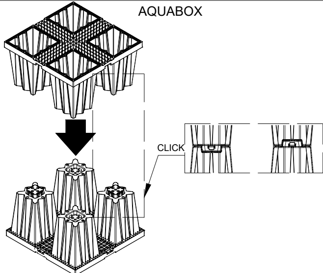
3 CONNETTORE SINGOLO
