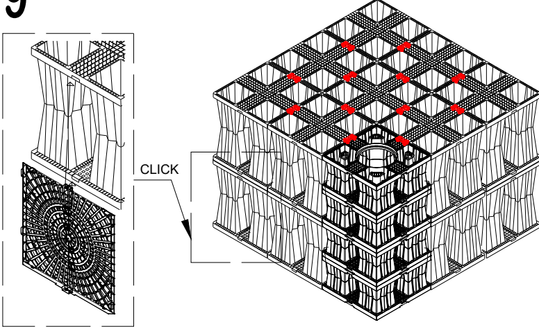
GRIGLIA LATERALE AQUABOX
