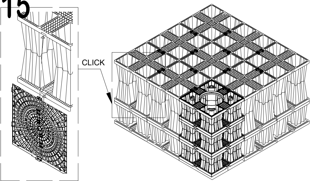
GRIGLIA LATERALE AQUABOX
