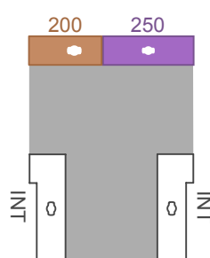
ÉPAISSEUR 250 mm
