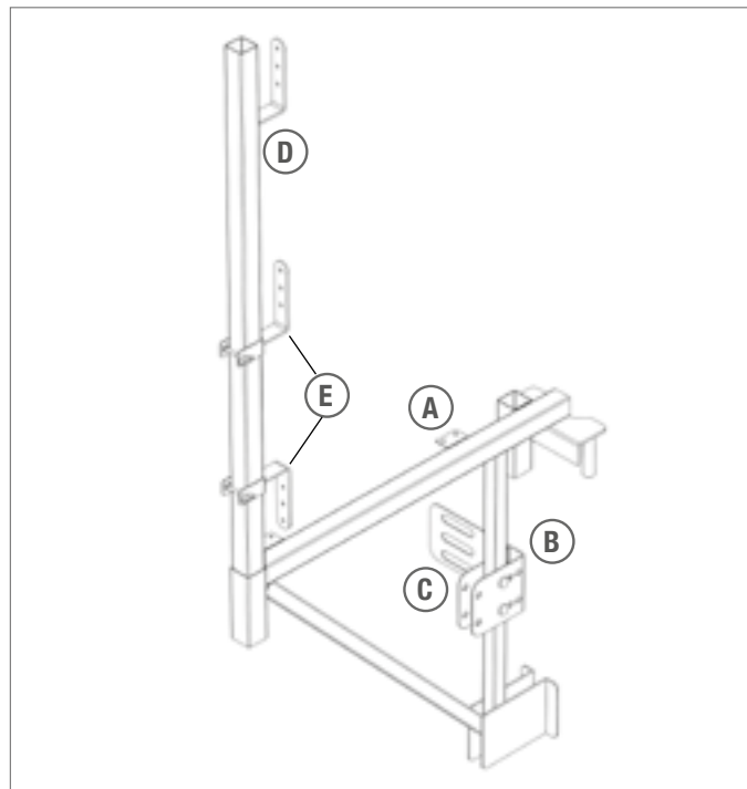
Garde-corps arrière
