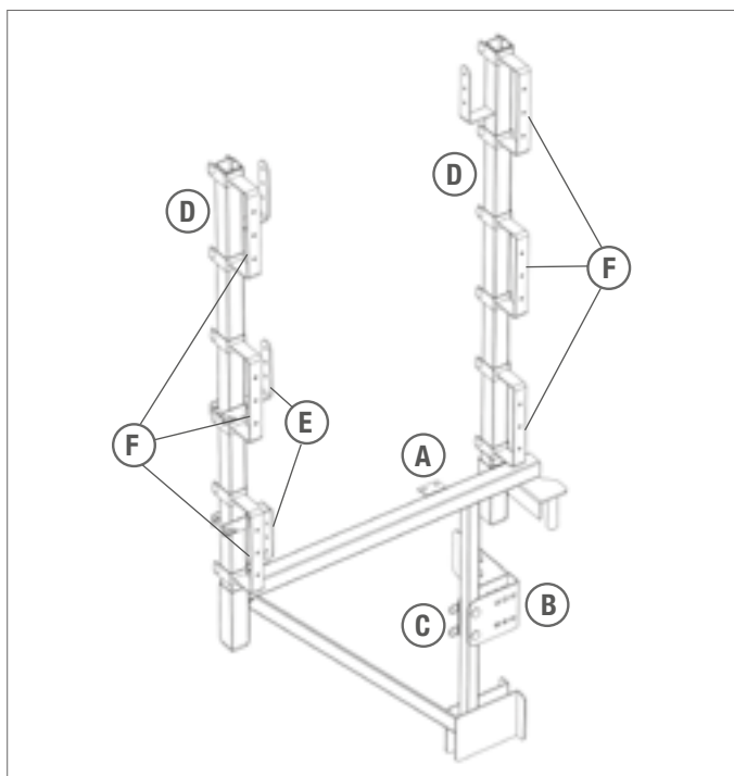
Garde-corps latéral
