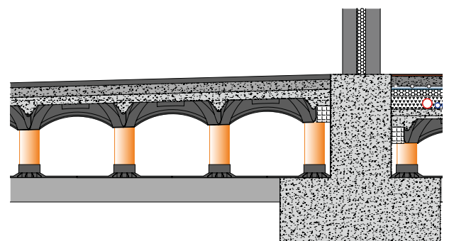
Rampe à pente finie
