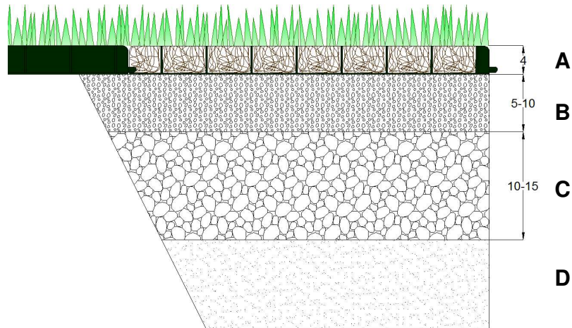
A- Salvaverde A; B- Couche de pose; C- Couche portante; D- Sol existant
