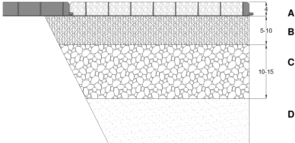
A- Salvaverde A; B- Couche de pose; C- Couche portante; D- Sol existant
