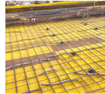
② COLOCACIÓN ENCOFRADO INFERIOR Y ZONAS MACIZAS
