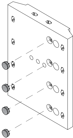
1. GEOPANEL CL HANDLE CAPS ROMOVING RIMOZIONE TAPPI MANIGLIE DEL GEOPANEL CL
