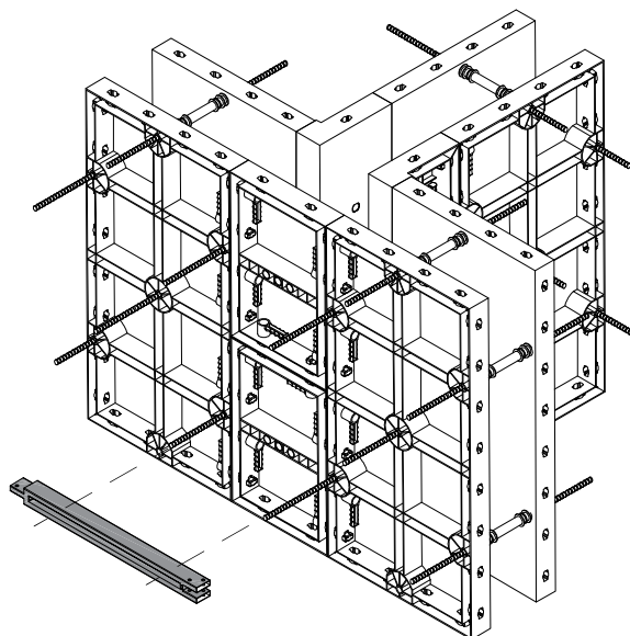
10. ALIGNMENT BARS INSTALLATION INSTALLAZIONE BARRE ALLINEATRICI
