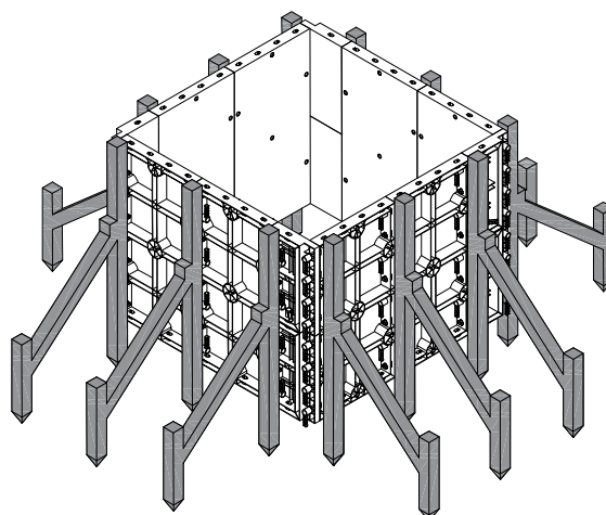
4. PICKETS SUPPORTS INSTALLATION INSTALLAZIONE SUPPORTI PER PICCHETTI
