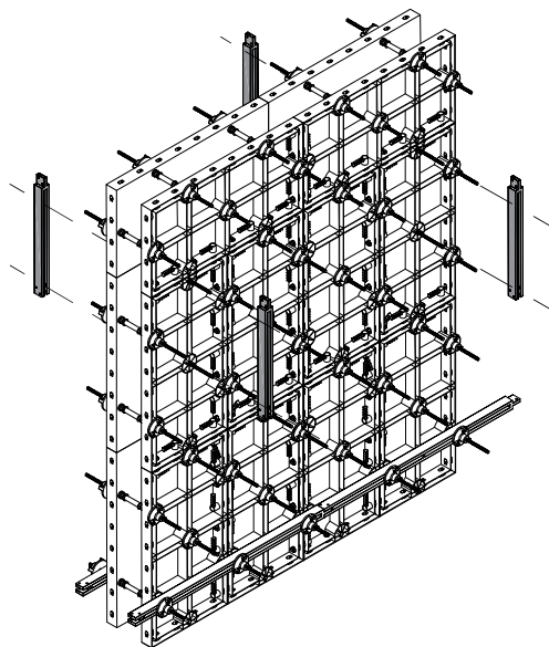
3. ANCHOR NUTS INSTALLATION INSTALLAZIONE ROSETTE
