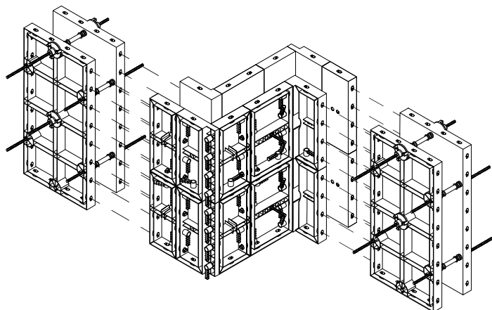
9. ALIGNMENT BARS INSTALLATION INSTALLAZIONE BARRE ALLINEATRICI
