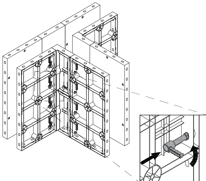
9. INTERNAL CORNERS POSITIONING POSIZIONAMENTO ANGOLI INTERNI
