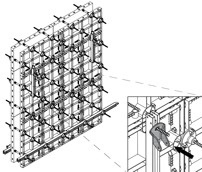
4. PUSH/PULL PROP INSTALLATION INSTALLAZIONE PUNTELLO
