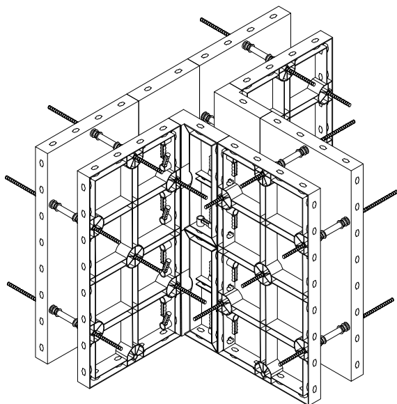
9. INTERNAL CORNERS POSITIONING POSIZIONAMENTO ANGOLI INTERNI
