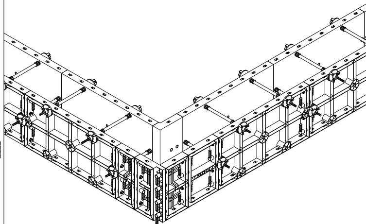
2. WALL ASSEMBLING ASSEMBLAGGIO MURI
