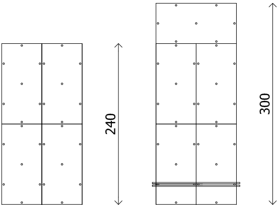
14. GENERAL DISTRIBUTION OF ALIGNMENT BARS DISTRIBUZIONE GENERALE DELLE BARRE ALLINEATRICI
