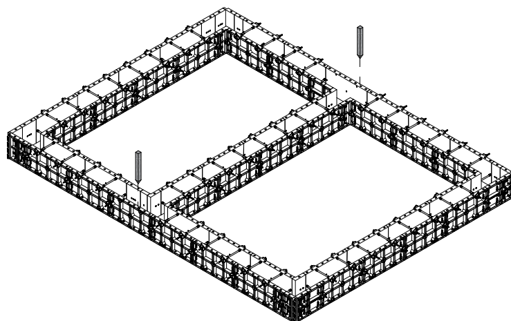
3. PICKETS INSTALLATION INSTALLAZIONE PICCHETTI
