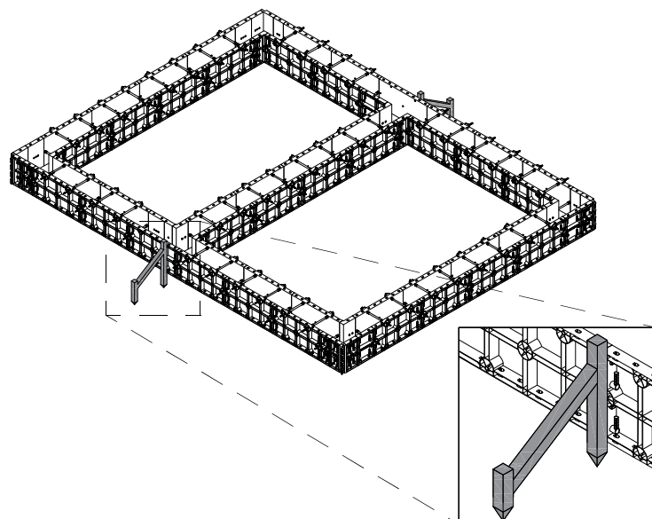
4. PICKETS SUPPORTS INSTALLATION INSTALLAZIONE SUPPORTI PER PICCHETTI
